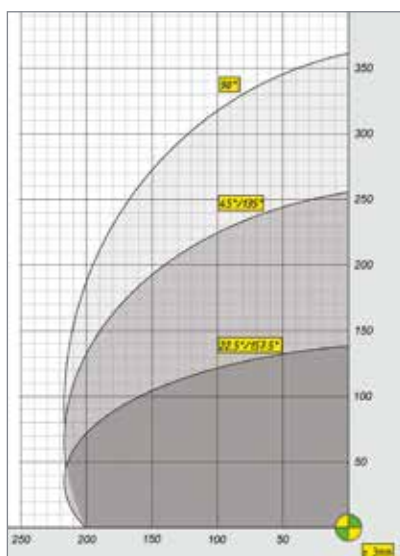
SW 553 - lama / blade \varnothing 550 mm
