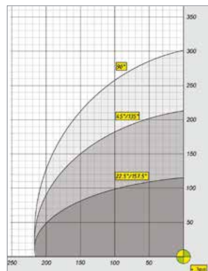
SW 553-R - lama / blade \varnothing 550 mm
